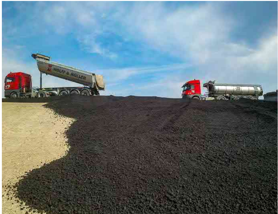
Aufbringen der Tragschicht
